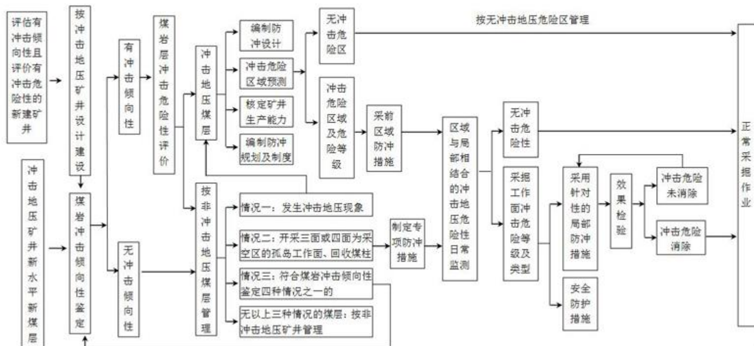
防治煤矿冲击地压基本流程示意图
